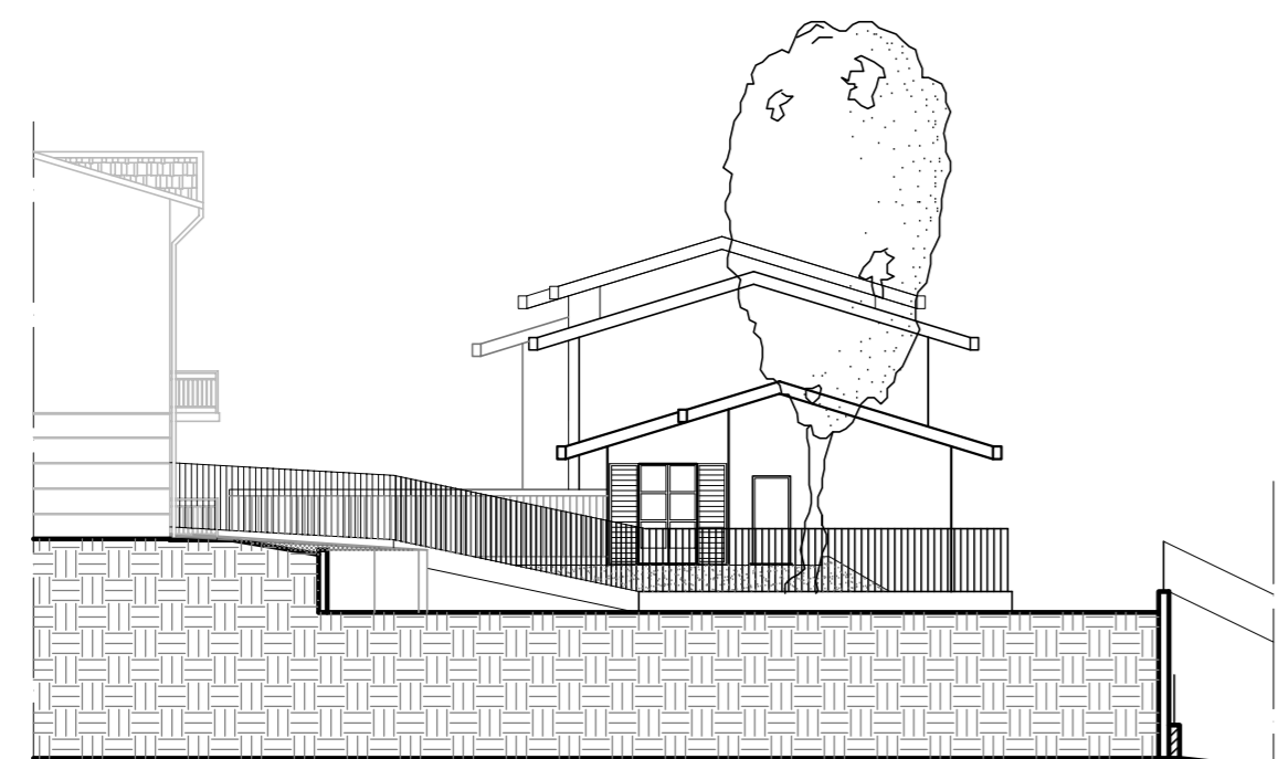
PROSPETTO OVEST
