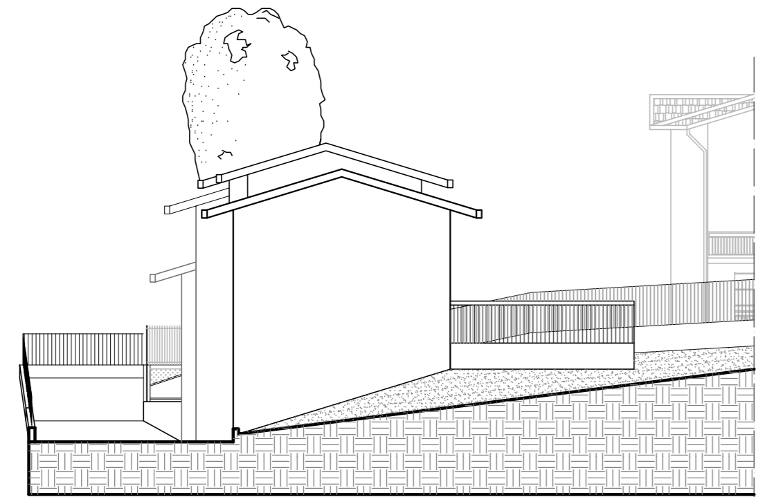
PROSPETTO EST
