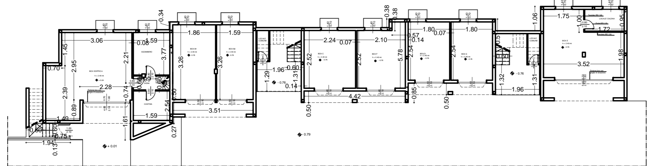
PIANTE PIANO INTERRATO
