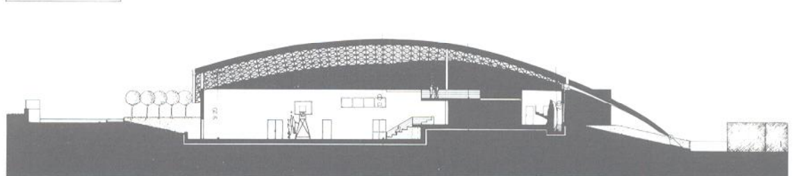
SEZIONE Y-Y
