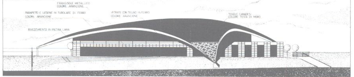
PROSPETTO EST
