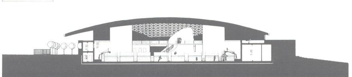
SEZIONE X-X
