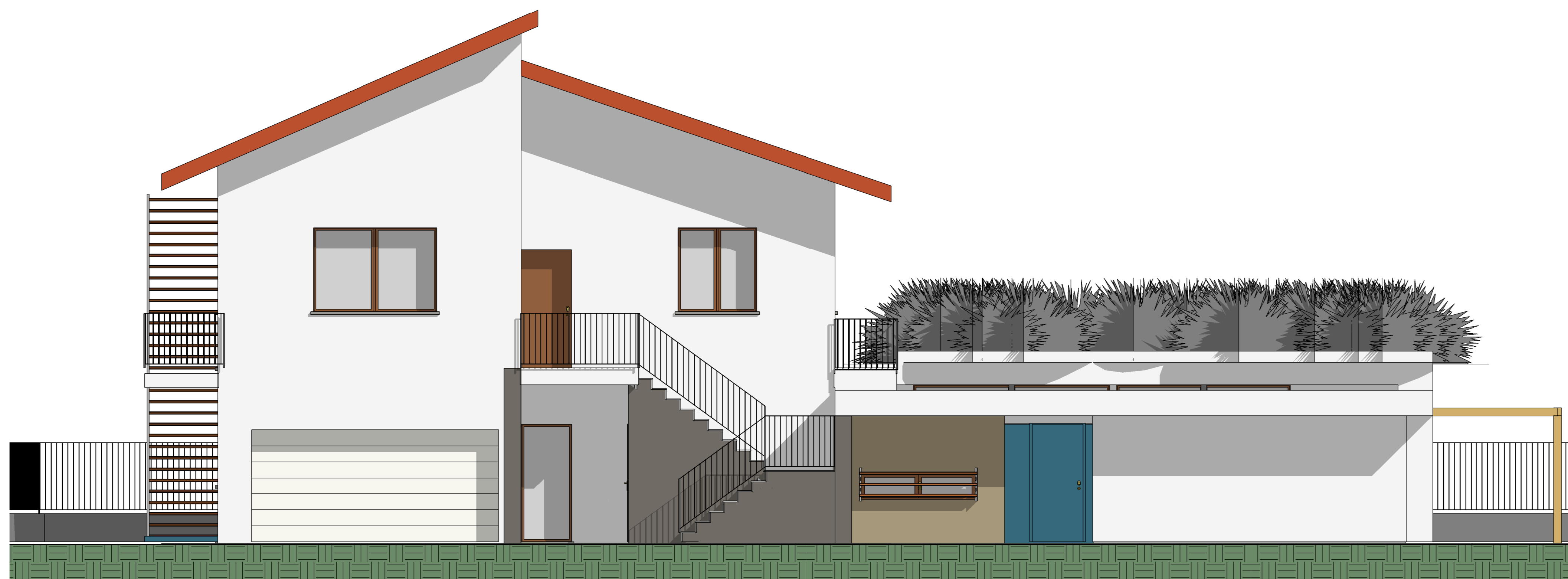
PROSPETTO FRONTALE
