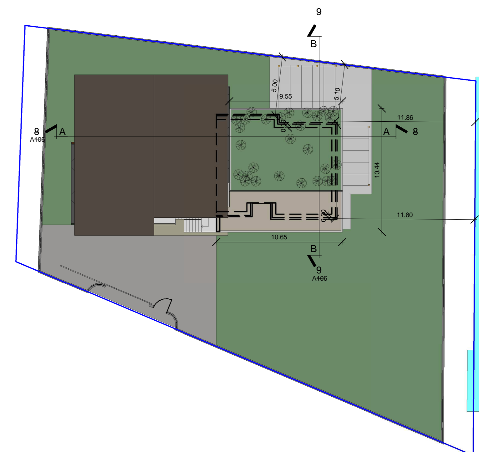
PLANIMETRIA GENERALE
